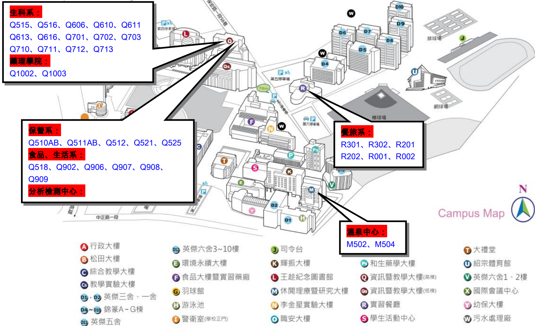
圖五之三、嘉藥學校財團法人嘉南藥理大學 校區作業環境監測平面配置圖
